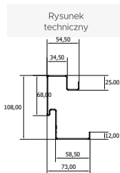
Ciepły próg PVC/ALU z przegrodą termiczną Prestige, Optimum
