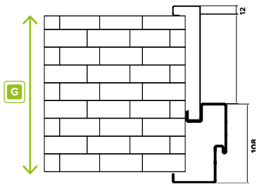
Portal z ościeżnicą wewnętrzną IRON
