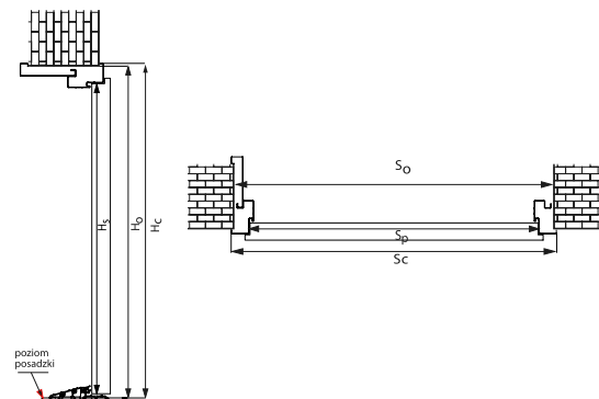
Wymiarowanie drzwi IRON z ościeżnicą regulowaną
