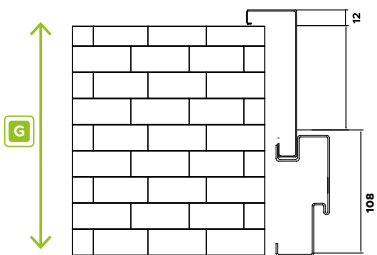
Opaska z ościeżnicą wewnętrzną IRON
