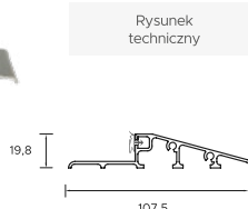
Próg aluminiowy z uszczelką Premium, Normal, Protect, Iron do ościeżnicy "9" (kątovej), "11" (wewnętrznej)
