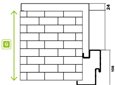
Portal z ościeżnicą regulowaną IRON
