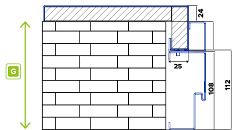
Opaska z ościeżnicą wewnętrzną IRON
