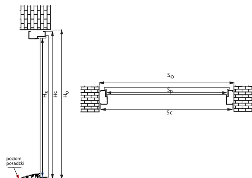
Wymiarowanie drzwi IRON z ościeżnicą symetryczną
