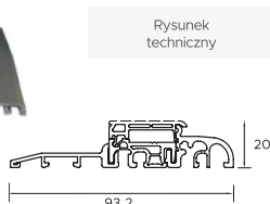
Ciepły próg PVC/ALU z przegrodą termiczną Alu Hybrid
