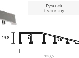
Próg aluminiowy Optimum,
