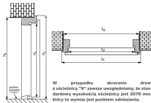
Wymiarowanie drzwi IRON z ościeżnicą kątową
