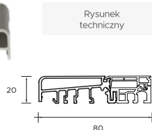
Ciepły próg PVC/ALU z przegrodą termiczną Prestige, Optimum
