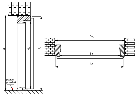
Wymiarowanie drzwi z ościeżnicą „11”, „12”, aluminiowo-kompozytową oraz TERMO i TERMO PRESTIGE LUX
