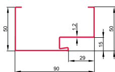
OŚCIEŻNICA FD/25/21/B/40
