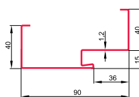
OŚCIEŻNICA FD/21/C
