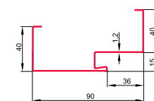
OŚCIEŻNICA FD/21/C
