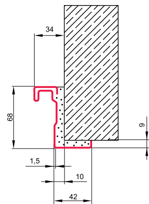
OŚCIEŻNICA EI30
