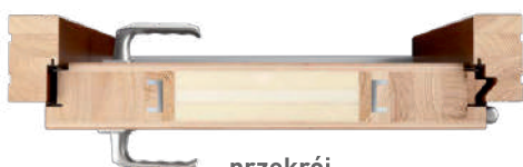
przekrój drzwi przylgowych 78 mm THERMO WOOD
