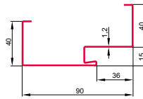
OŚCIEŻNICA FD/21/C
