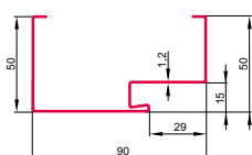
OŚCIEŻNICA FD/25/21/B/40
