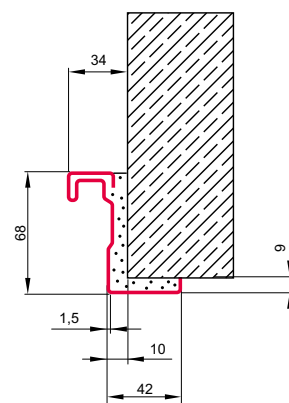
OŚCIEŻNICA EI30
