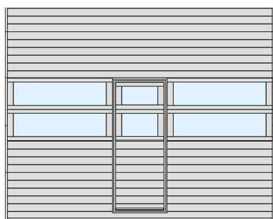
BRAMY Z DRZWIAMI PRZEJŚCIOWYMI I PANELAMI Z SEKCJĄ ALUMINIOWĄ PRZESZKLONĄ
