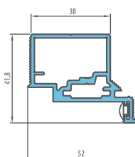
PRZEKRÓJ OŚCIEŻNICY ALUMINIOWEJ
