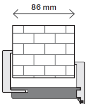
ZAKRES MINIMALNY regulacja po skróceniu pióra kątownika
