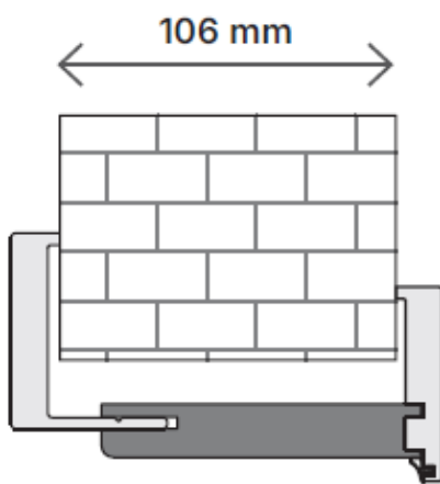
ZAKRES STANDARDOWY regulacja bez skróconego pióra kątownika
