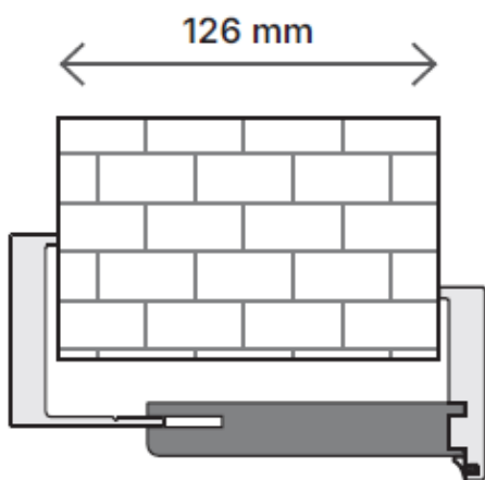
ZAKRES MAKSYMALNY regulacja bez skróconego pióra kątownika
