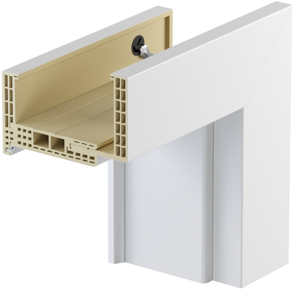
Przekrój ościeżnicy odwrotna przylga
